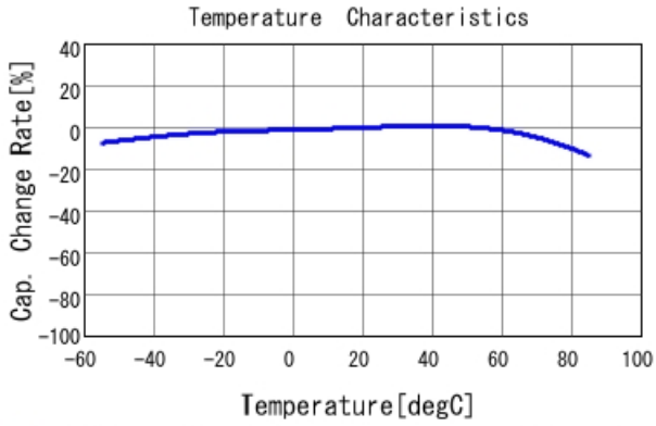
■ GRM153R60J225ME95 C-Temp. capchange, DCO. 0V, ACO. 2Vrm
