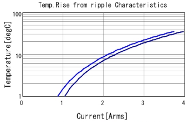
GRM153R60J225ME95 Temp. rise ■ 500kHz ■ 1MHz
