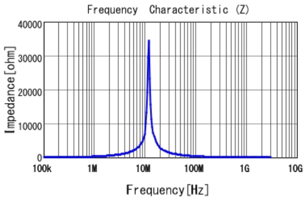
1273AS-H-470M |Z|
