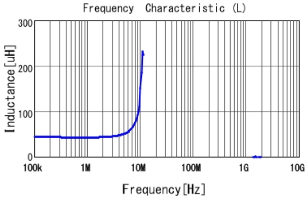
1273AS-H-470M L
