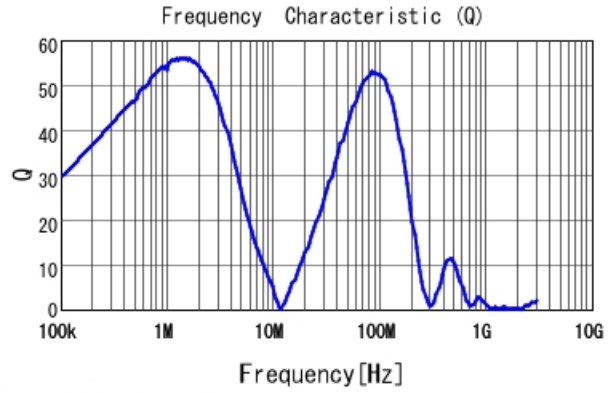
1273AS-H-470M Q
