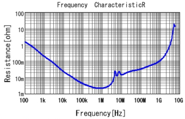
GRM32DR11E475KA61 R DCOV, 20degC
