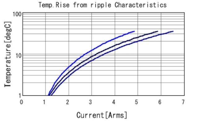
GRM32DR11E475KA61 Temp. rise — 100kHz — 500
