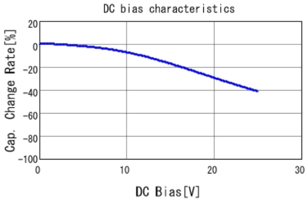
GRM32DR11E475KA61 C-DC bias capchange, 20.0degC, A
