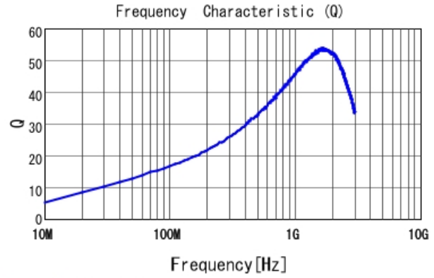
LQG15WZ10NJ02 Q
