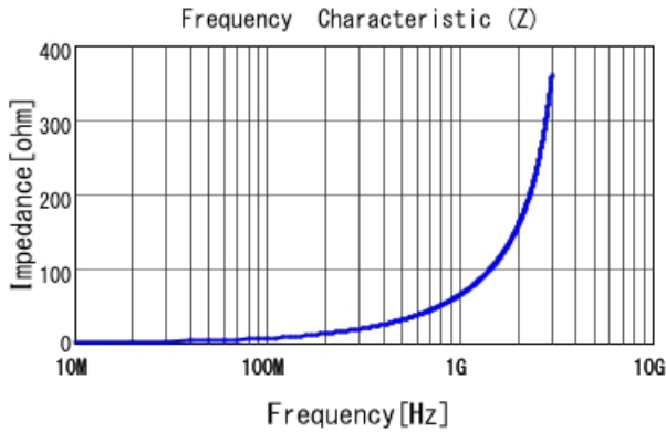
LQG15WZ10NJ02 |Z|
