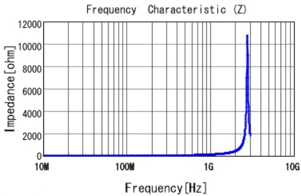
LQG15HH18NJ02 |Z|
