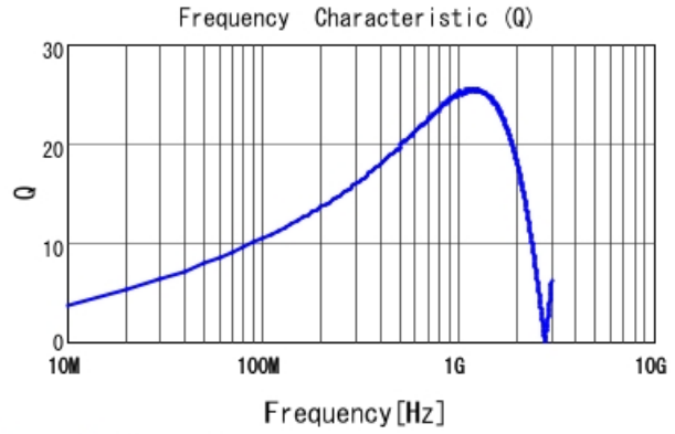
LQG15HH18NJ02 Q
