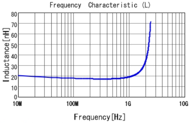
LQG15HH18NJ02 L
