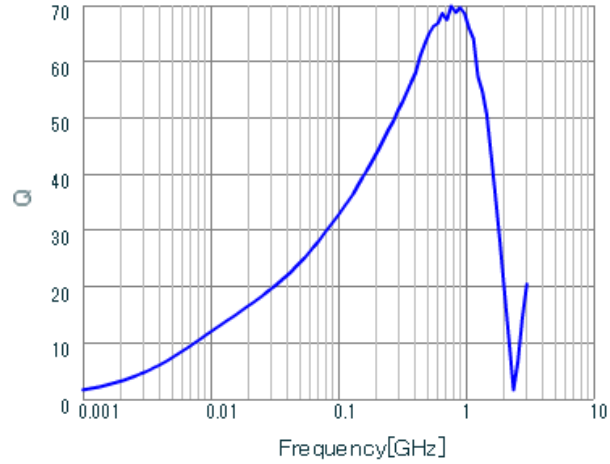
LQW18AN78NG8Z Q.
