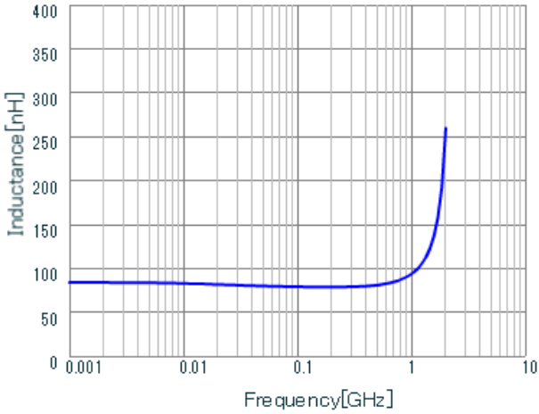
LQW18AN78NG8Z L.
