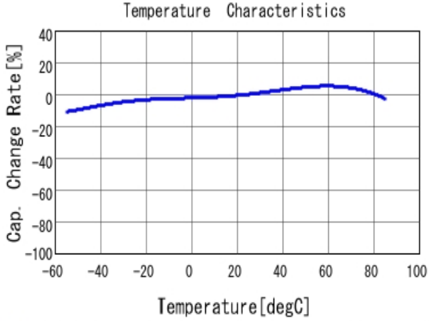
■ GRM32ER61A476KE20 C-Temp. capchange, DCO. 0V, ACO. 5Vrm
