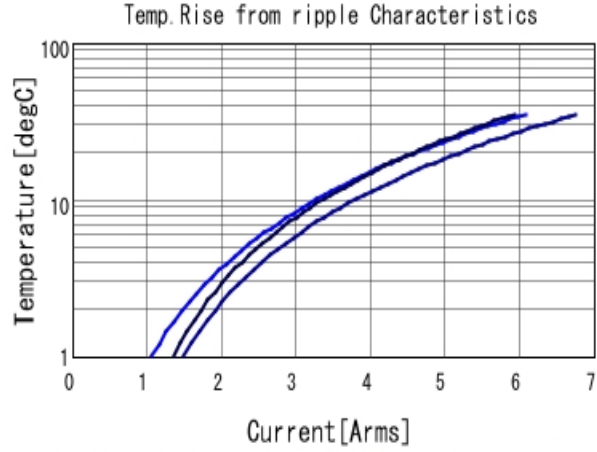
GRM32ER61A476KE20 Temp. rise ■ 60kHz ■ 300kHz ■ 600kHz
