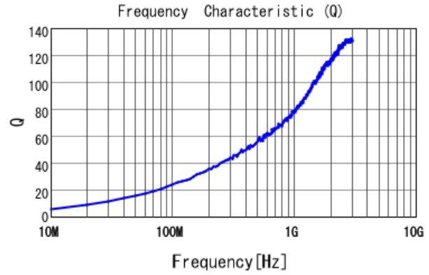
LQW15AN2N4D10 Q
