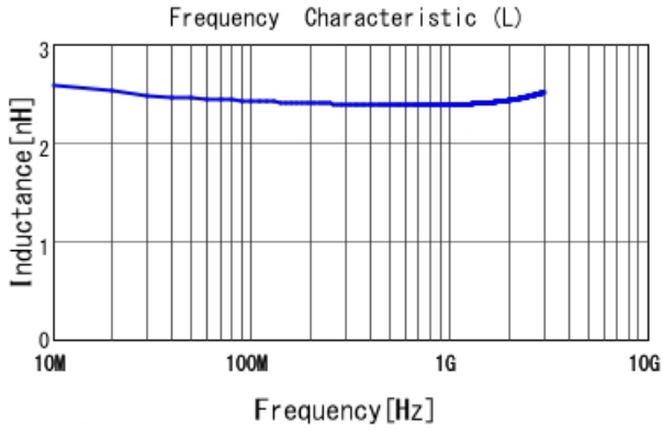
LQW15AN2N4D10 L
