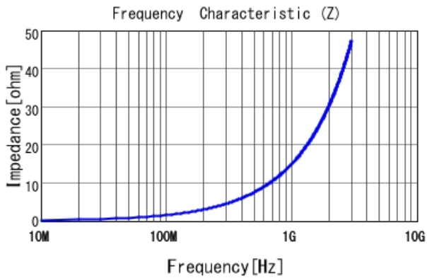
LQW15AN2N4D10 |Z|
