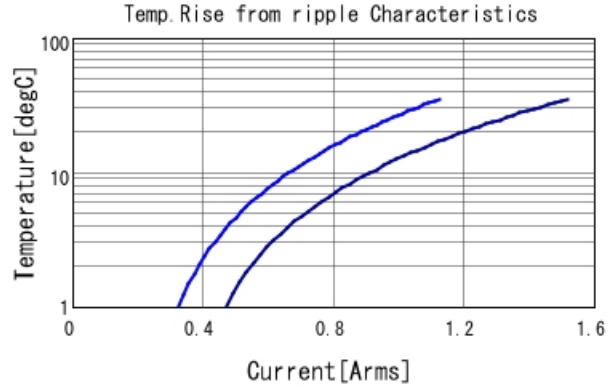
GRM155R71A104KA01 Temp. rise — 500kHz — 1MHz
