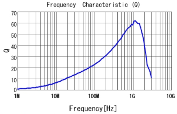
LQW15AN43NJ80 Q
