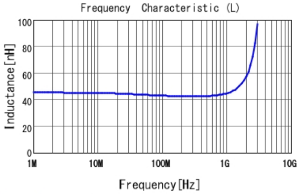
LQW15AN43NJ80 L
