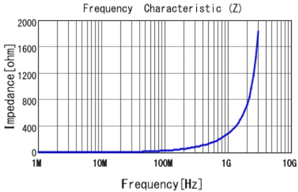
LQW15AN43NJ80 |Z|
