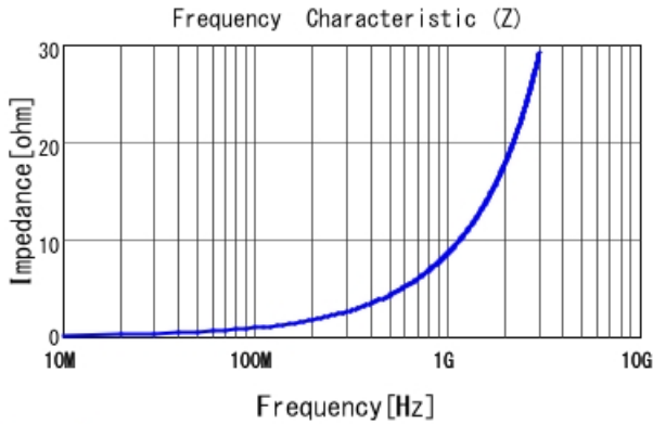
LQG15HH1N5C02 |Z|
