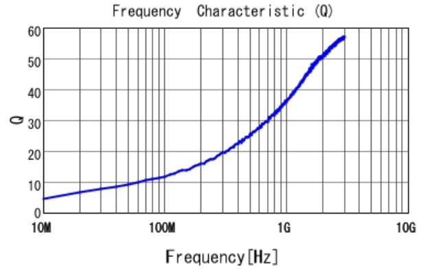
LQG15HH1N5C02 Q
