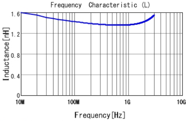
LQG15HH1N5C02 L
