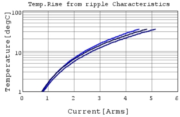
GCJ31CC71E106KA15 Temp.rise — 80kHz
