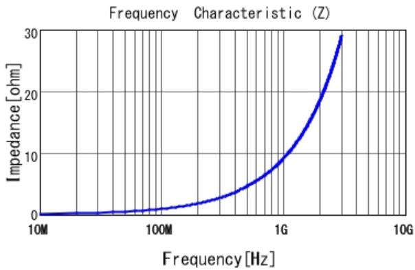
LQG15HN1N5S02 |Z|
