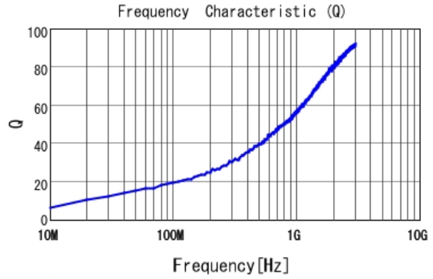
LQG15HN1N5S02 Q
