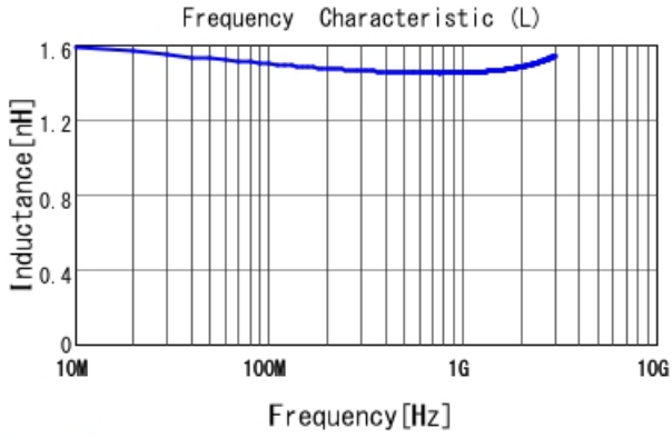
LQG15HN1N5S02 L
