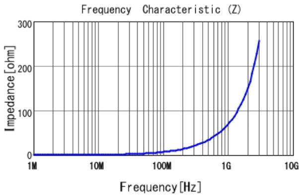
LQW15AN11NG8Z |Z|
