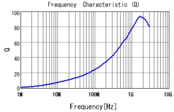
LQW15AN11NG8Z Q
