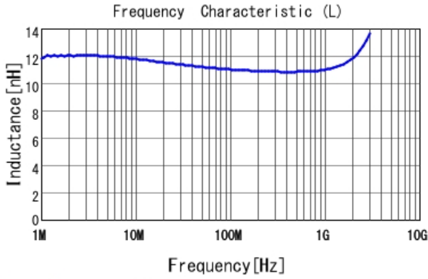
LQW15AN11NG8Z L
