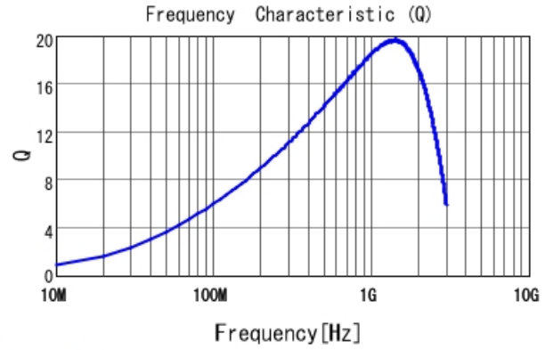
LQP03TG15NH02 Q
