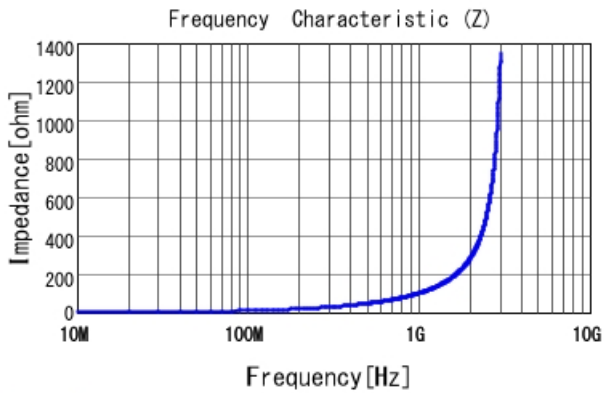
LQP03TG15NH02 |Z|
