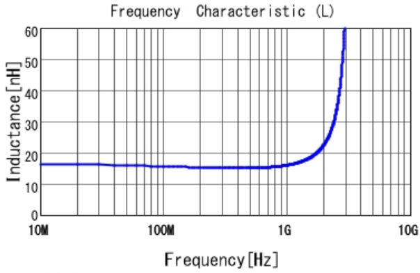
LQP03TG15NH02 L
