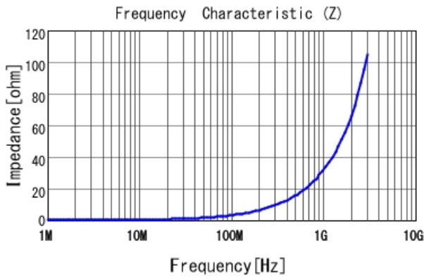
LQW15AN5N2G8Z |Z|
