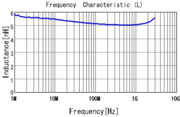
LQW15AN5N2G8Z L
