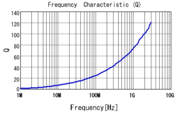
LQW15AN5N2G8Z Q
