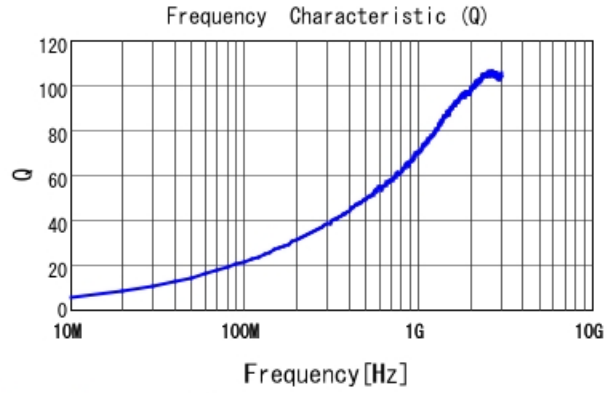
LQW15AN5N6D1Z Q
