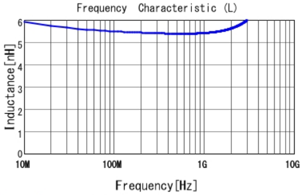
LQW15AN5N6D1Z L
