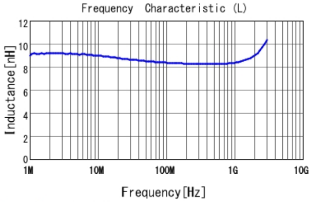
LQW15AN8N3G8Z L
