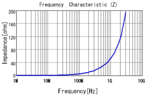
LQW15AN8N3G8Z |Z|
