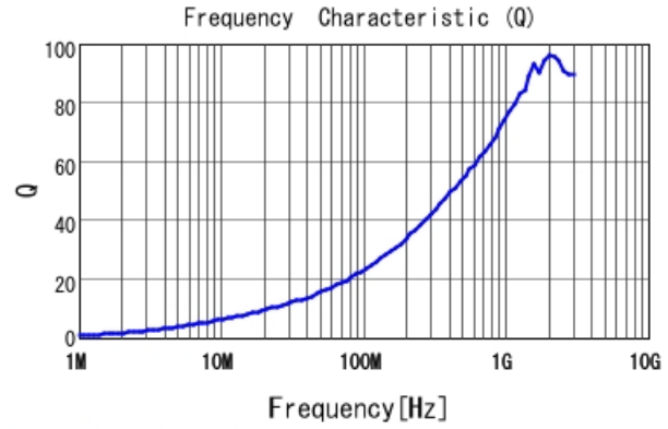
LQW15AN8N3G8Z Q
