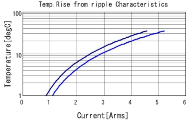
GRM21BR61H475ME51 Temp. rise ■ 500kHz ■ 1MHz
