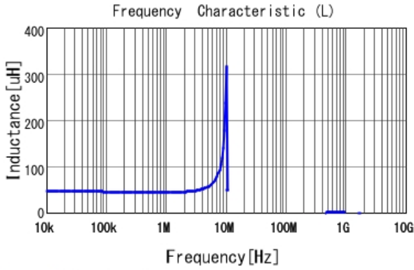
#B952AS-H-470M=P3 L
