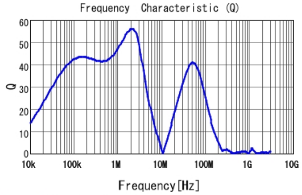
#B952AS-H-470M=P3 Q
