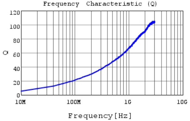
LQW15AN6N8H00 Q
