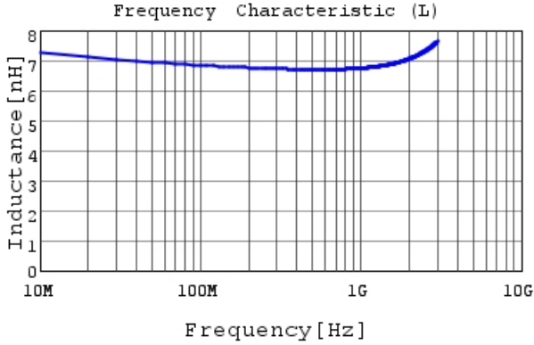
LQW15AN6N8H00 L
