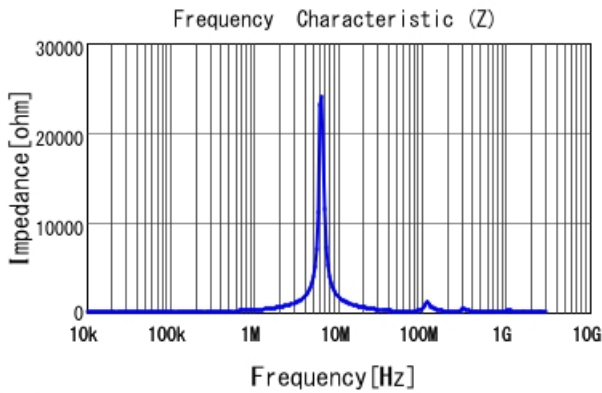
■ MDH12577C-470MA |Z|
