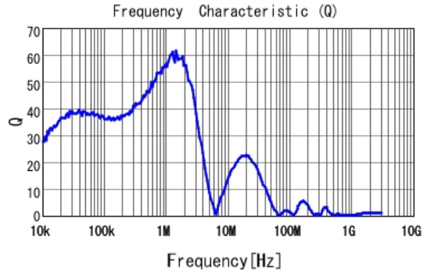
■ MDH12577C-470MA Q
