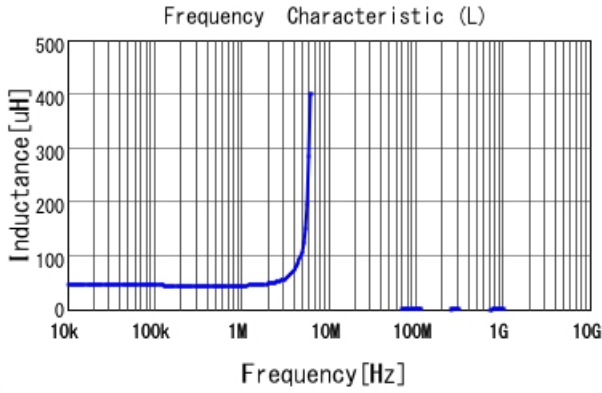
■ MDH12577C-470MA L
