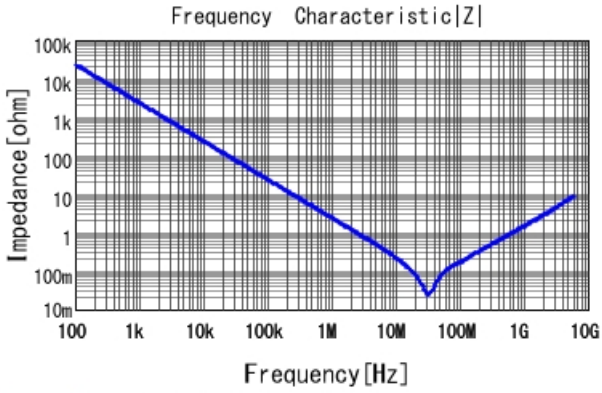
GRM155R71E683KE14 |Z| DCOV, 25degC
