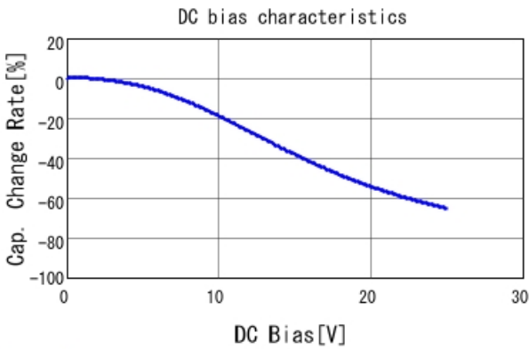
GRM155R71E683KE14 C-DC bias capchange, 25.0degC, A
