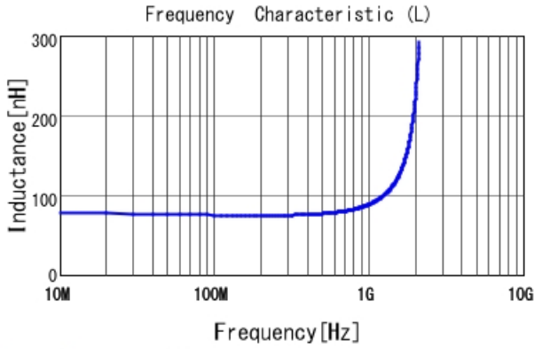
LQW18AN75NG0Z L
