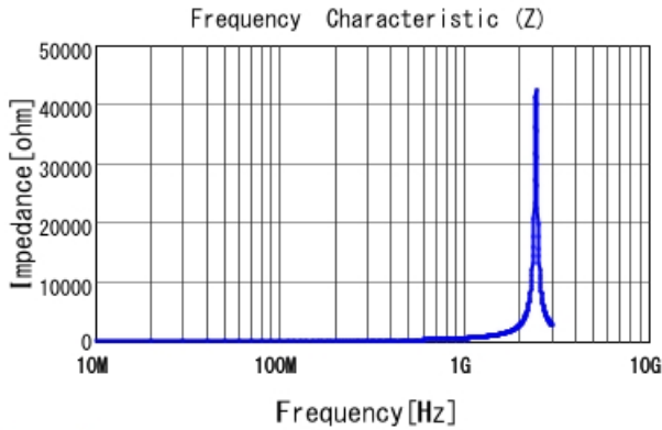
LQW18AN75NG0Z |Z|
