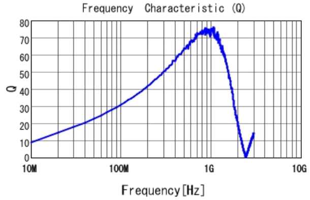
LQW18AN75NG0Z Q
