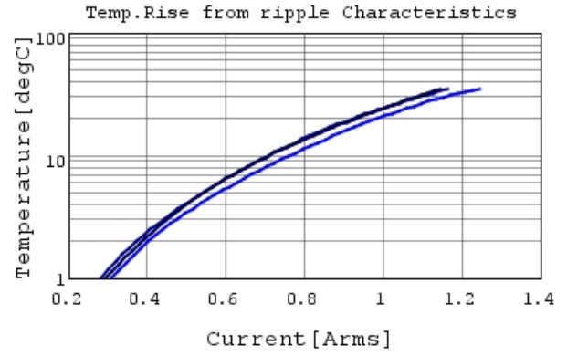
GQM22M5C2H120JB01 Temp.rise 500MHz
