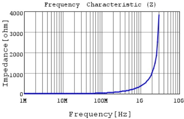
LQW15AN56NG80 |Z|
