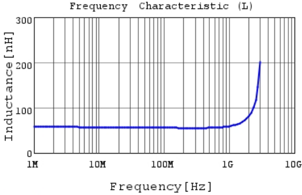
LQW15AN56NG80 L
