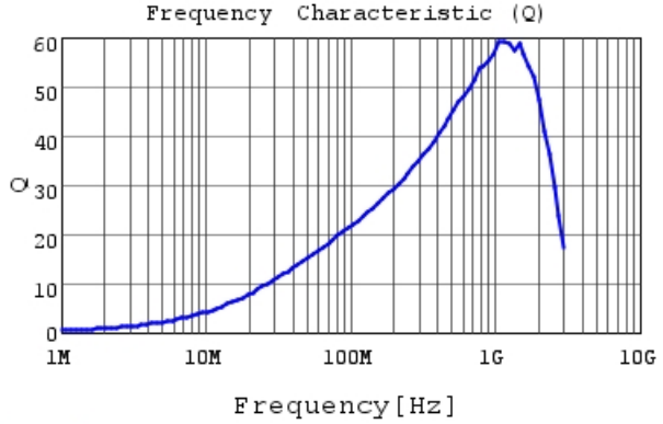
LQW15AN56NG80 Q
