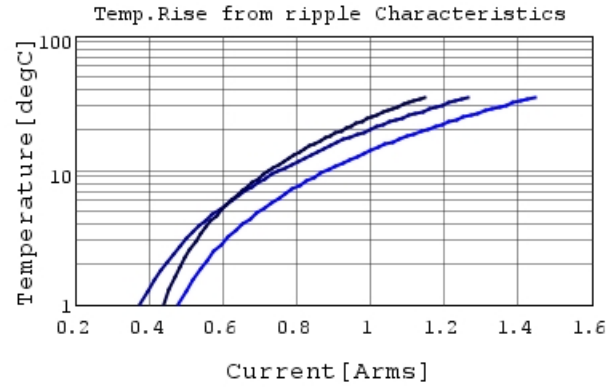
GJM0335C1E330JB01 Temp.rise 400MHz
