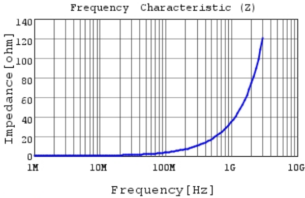
LQW15AN5N7C8Z |Z|
