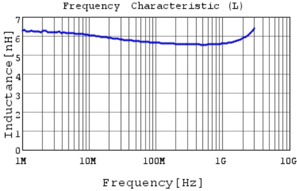
LQW15AN5N7C8Z L
