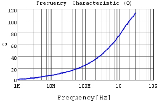
LQW15AN5N7C8Z Q
