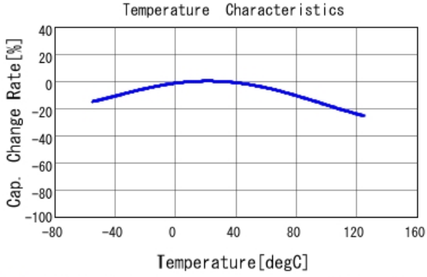
■ GRM188D70J106MA73 C-Temp. capchange, DCO. 0V, ACO. 2Vrm
