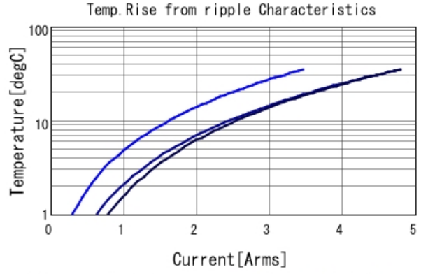
GRM188D70J106MA73 Temp. rise ■ 80kHz ■ 400kHz ■ 800kHz
