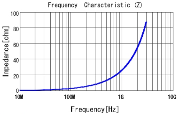
LQW15AN4N2C10 |Z|
