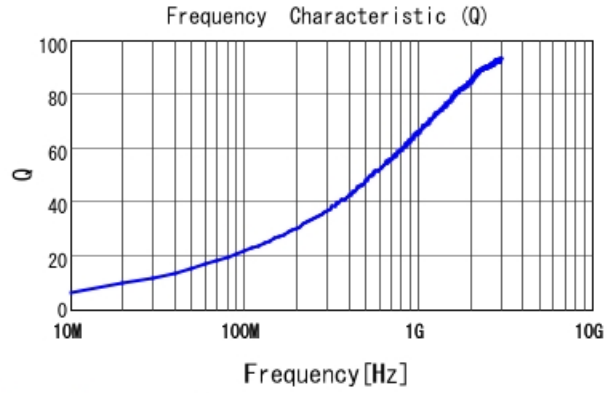
LQW15AN4N2C10 Q
