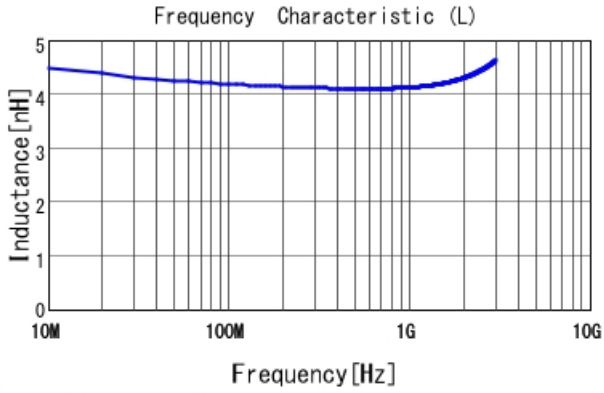
LQW15AN4N2C10 L
