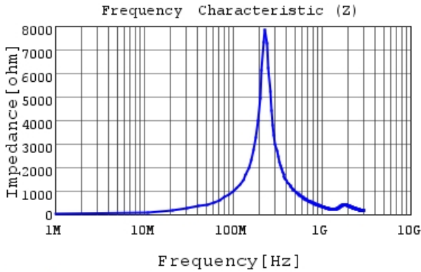
LQW15CN1R5M10 |Z|
