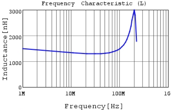
LQW15CN1R5M10 L
