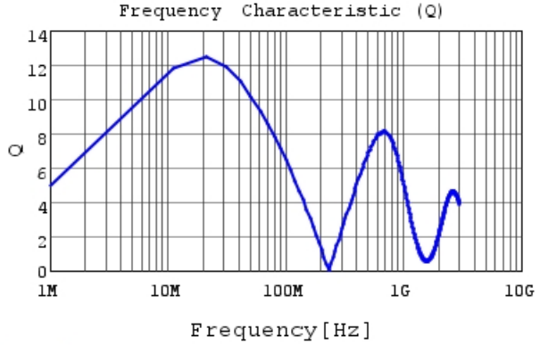
LQW15CN1R5M10 Q
