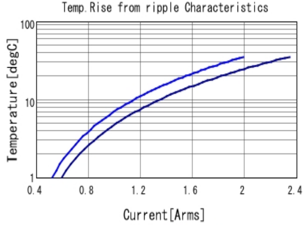
GRM155R60J334KE01 Temp. rise ■ 500kHz ■ 1MHz
