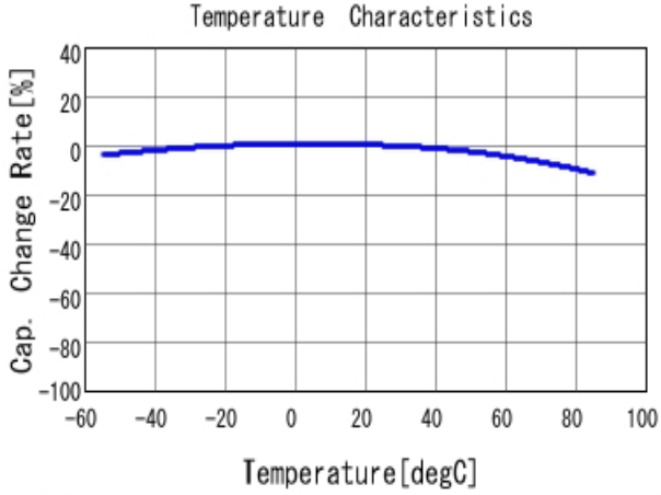
■ GRM155R60J334KE01 C-Temp. capchange, DCO. 0V, ACO. 5V rm
