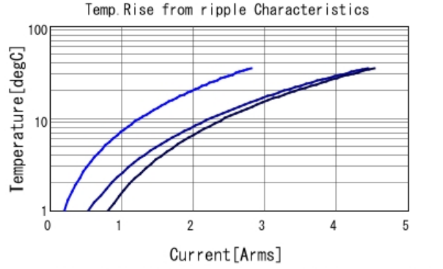
GRM21BR61E475KA12 Temp. rise — 100kHz — 500
