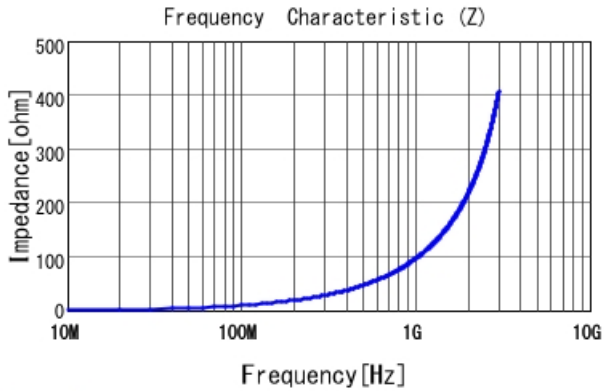
LQW18AS15NG0C |Z|
