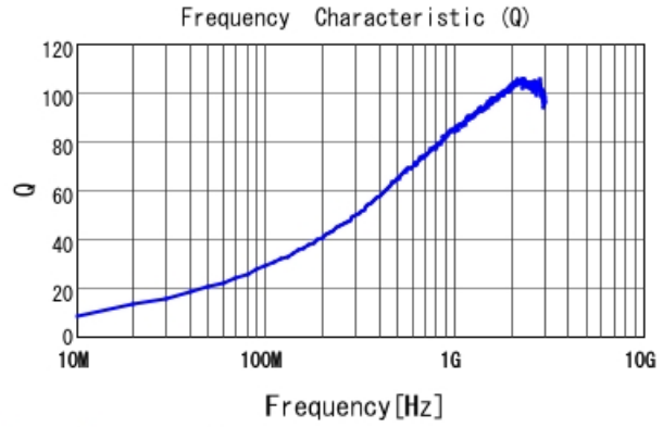
LQW18AS15NG0C Q
