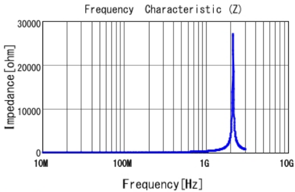
LQG15WZ43NG02 |Z|
