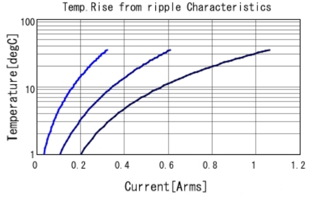
GRM43DR73A473KW01 Temp. rise ■ 30kHz ■ 100kHz ■ 300kHz
