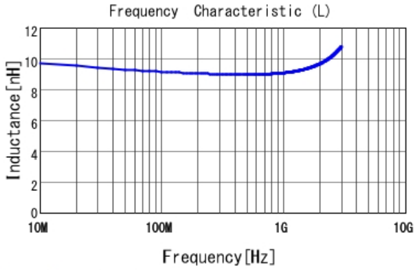
LQW15AN9N2J00 L
