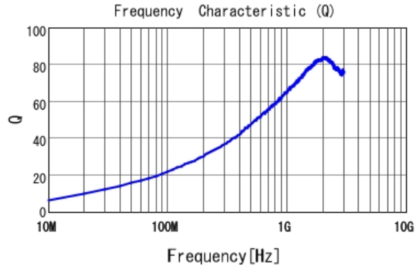
LQW15AN9N2J00 Q
