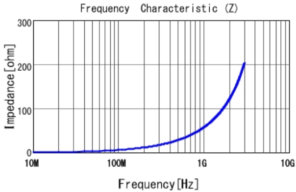
LQW15AN9N2J00 |Z|
