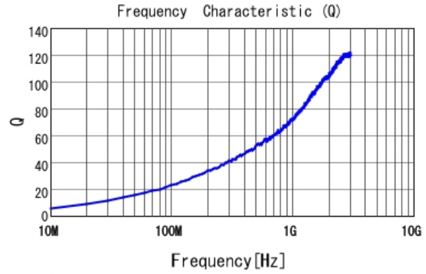
LQW15AN3N3D10 Q
