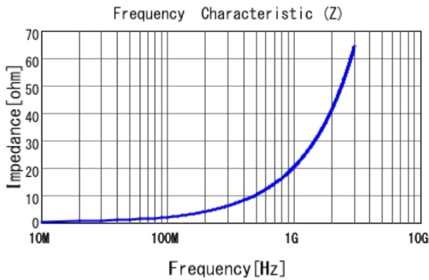
LQW15AN3N3D10 |Z|
