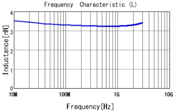
LQW15AN3N3D10 L
