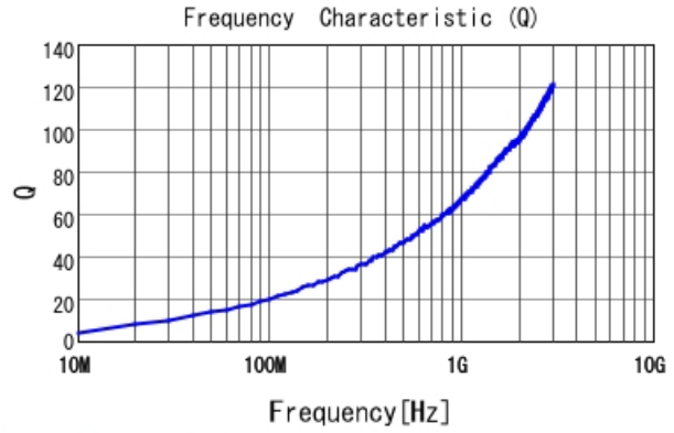
LQW15AN2N7D00 Q
