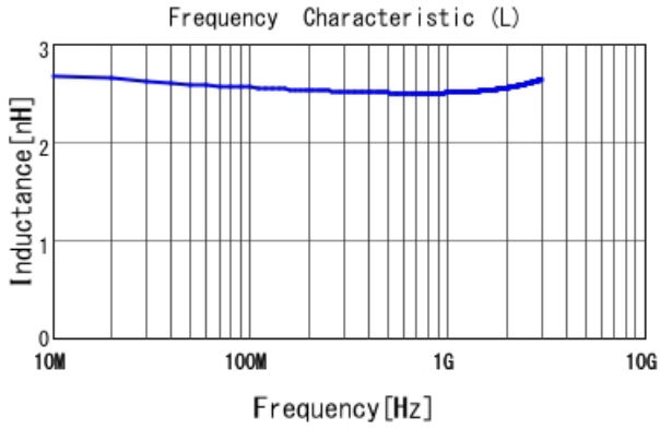
LQW15AN2N7D00 L
