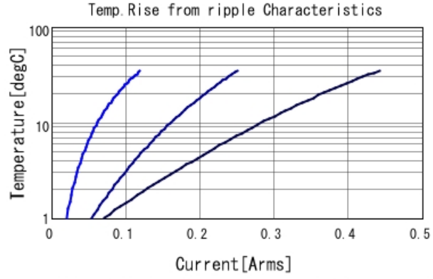
GRM21BR72E153KW03 Temp. rise — 30kHz — 100kHz
