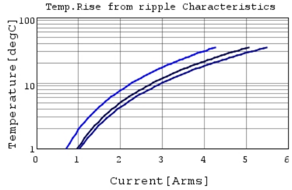
GCM31CC71H475KA03 Temp.rise — 100kHz —
