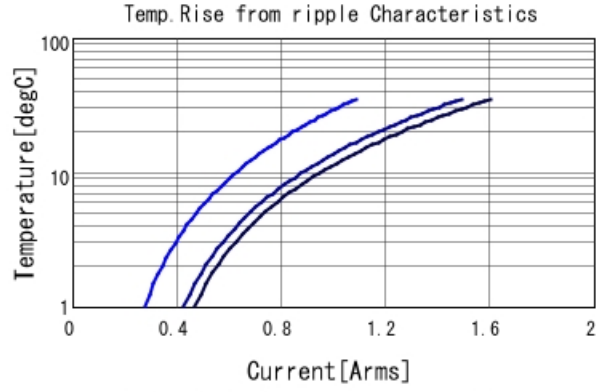
GCM188R71C104KA37 Temp. rise — 400kHz — 800I
