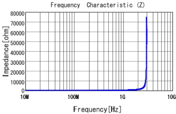
LQW15AW51NH80 |Z|
