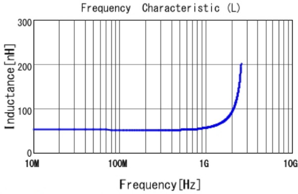
LQW15AW51NH80 L
