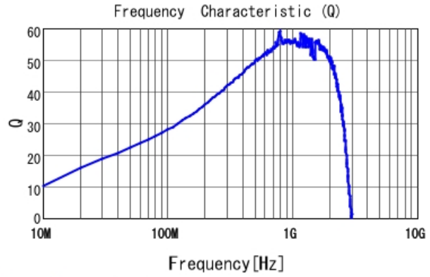
LQW15AW51NH80 Q
