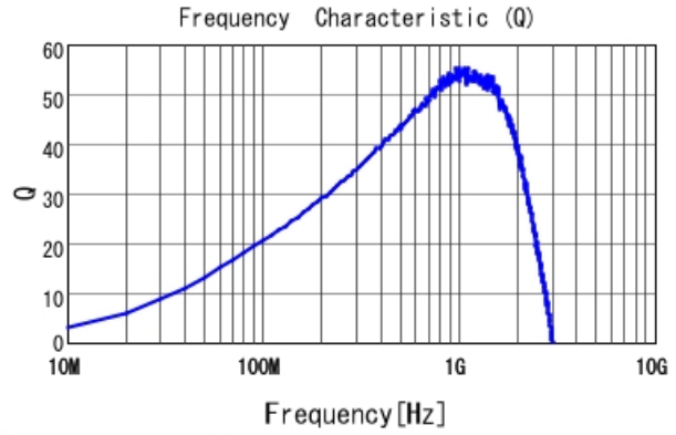
LQW15AN75NG00 Q
