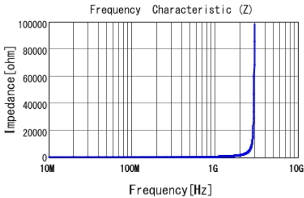
LQW15AN75NG00 |Z|
