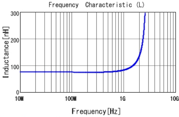
LQW15AN75NG00 L
