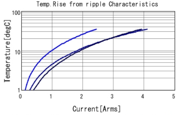
GRM21BR71E225KE11 Temp. rise ■ 100kHz ■ 500kHz ■ 1MHz
