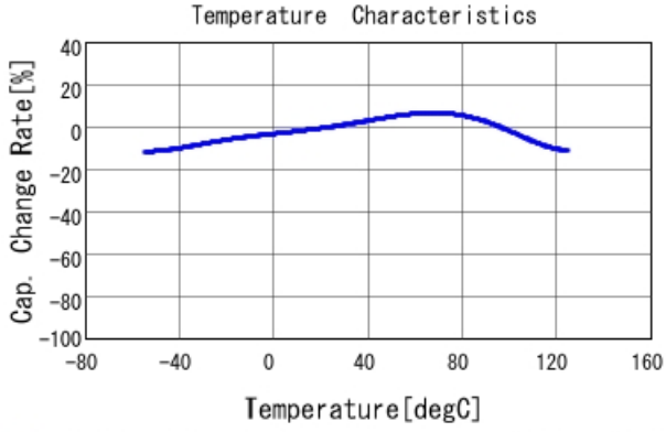
■ GRM21BR71E225KE11 C-Temp. capchange, DCO. 0V, ACO. 8Vrm
