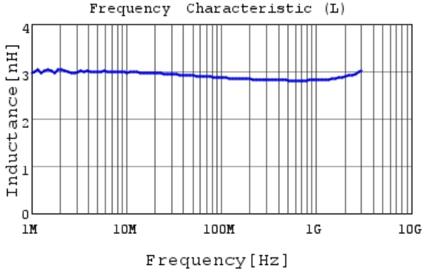
LQW15AN2N8G8Z L
