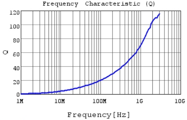
LQW15AN2N8G8Z Q
