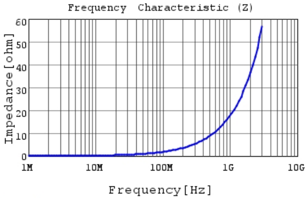
LQW15AN2N8G8Z |Z|
