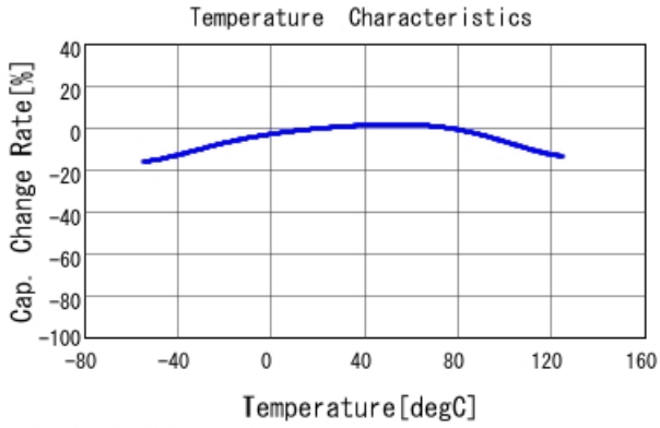
■ GRM033C71A104ME14 C-Temp. capchange, DCO. 0V, ACO. 2V rm
