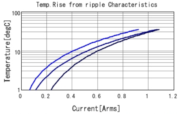
GRM033C71A104ME14 Temp. rise ■ 400kHz ■ 800kHz ■ 1MHz
