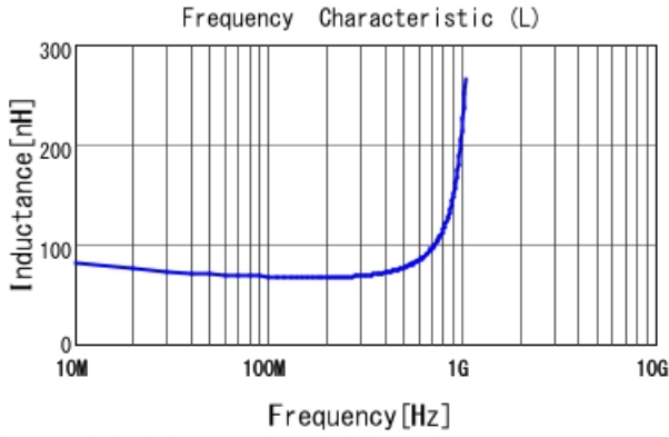
LQG15HZ68NH02 L
