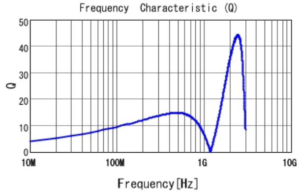
LQG15HZ68NH02 Q
