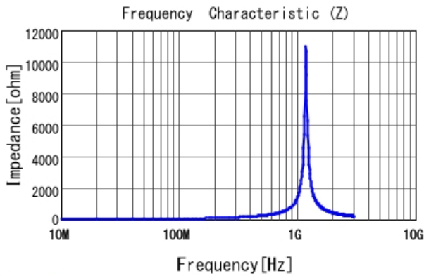
LQG15HZ68NH02 |Z|
