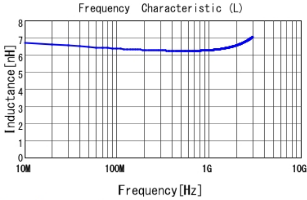
LQW15AN6N5D00 L
