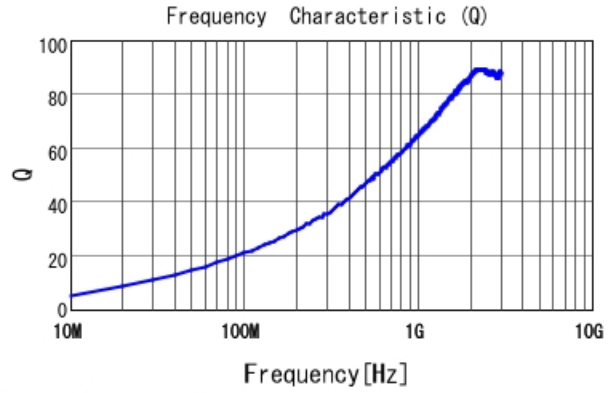
LQW15AN6N5D00 Q
