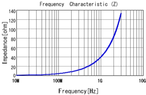
LQW15AN6N5D00 |Z|
