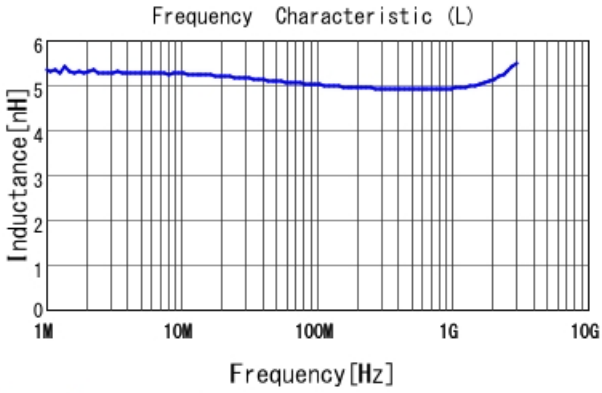
LQW15AN4N9B80 L
