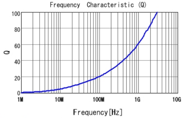
LQW15AN4N9B80 Q
