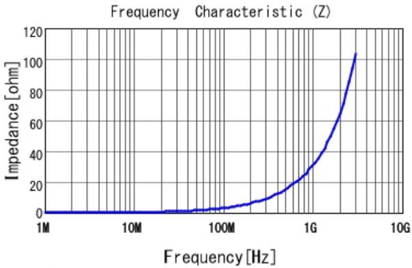
LQW15AN4N9B80 |Z|
